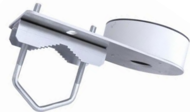
HIK134E + Z25DV75 + DS-1280ZJ-DM46
