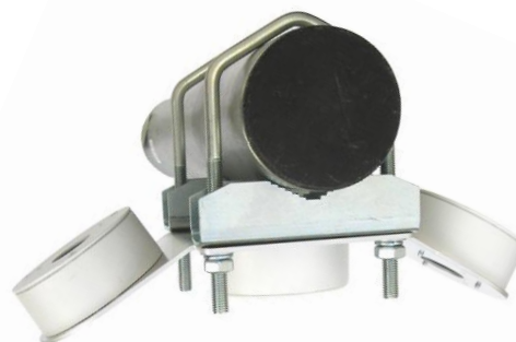
DAH100E TRIO + 2x Z5V105 montáž na trubku (Ø 90mm)
